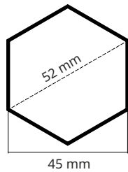
Querschnitt Standbein-Profil
