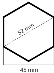
Querschnitt Standbein-Profil
