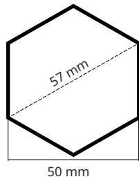
Querschnitt Standbein-Profil
