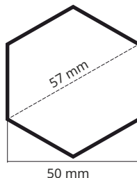
Querschnitt Standbein-Profil
