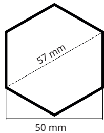
Querschnitt Standbein-Profil
