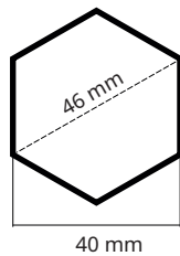
Querschnitt Standbein-Profil
